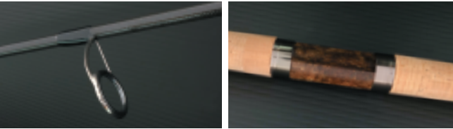
Rod Detail ガイドは過酷な釣行を考慮し、散逸してトルザイトではなくSiCチタンフレームKガイドを採用。リールシートはオリジナル・ウッズベアラーを採用、できるだけシンプルな形状に仕上げました。また、ブランクだけでなくガイドスレッドも黒で統一し、無駄の無いデザインにこだわりました
