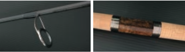
Rod Detail ガイドは過酷な釣行を考慮し、散逸してトルザイトではなくSiCチタンフレームKガイドを採用。リールシートはオリジナル・ウッズベアサーを採用、できるだけシンプルな形状に仕上げました。また、ブランクだけでなくガイドスレッドも黒で統一し、無駄の無いデザインにこだわりました
